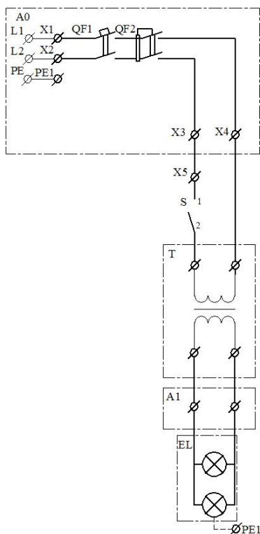
Электрическая схема 1
